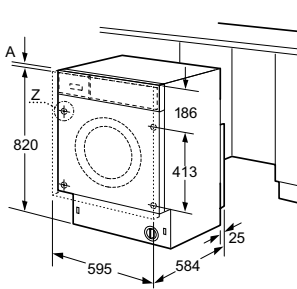
Posibilidad de colocación de la puerta del mueble con apertura hacia la derecha o izquierda
