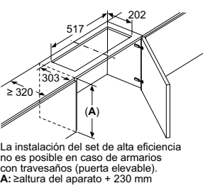
Montaje de la campana telescópica con set de alta eficiencia
