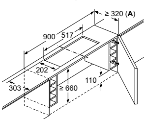
Montaje de la campana telescópica con set de alta eficiencia y marco de encastre
