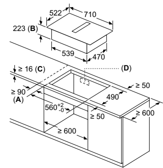
Placa combiInducción ED751HQ26E de 70 cm con extractor integrado
