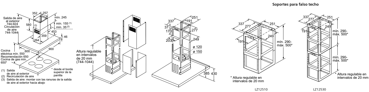
Set de recirculación de alta eficiencia para campana de isla
