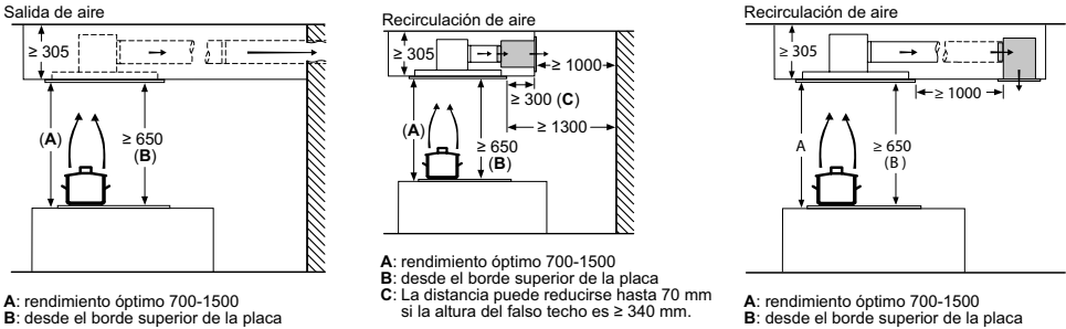
Sets de recirculación para extractor de techo LR97CBS20
