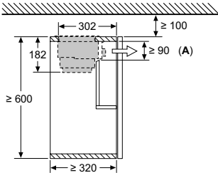
Montaje de la campana telescópica con set de alta eficiencia
