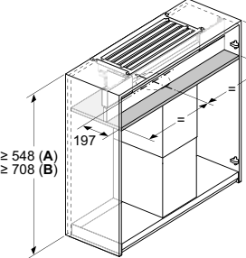
Montaje de la campana decorativa integrada con set de recirculación y prolongación de conducto
