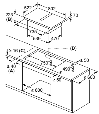
Placa flexInducción EX851HJ26E y combiInducción ED851HQ26E de 80 cm con extractor integrado en mueble de 80 cm
