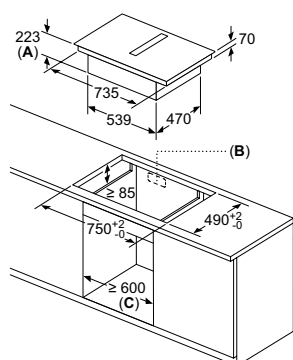
Placas flexInducción EX875LX67E, EX851HJ26E y combiInducción ED851HQ26E de 80 cm con extractor integrado en mueble de 60 cm
