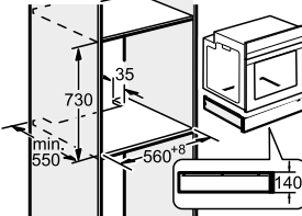
Instalación debajo de un horno de 60 cm
