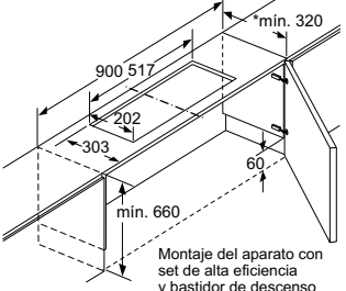
Montaje de la campana telescópica de 90 cm con set de alta eficiencia
