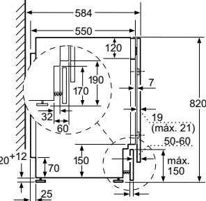
Posibilidad de colocación de la puerta del mueble con apertura hacia la derecha o izquierda
