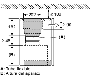
Montaje del módulo de integración con set de alta eficiencia
