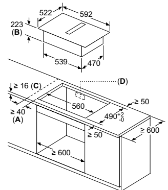
Placa combiInducción ED631HQ26E de 60 cm con extractor integrado
