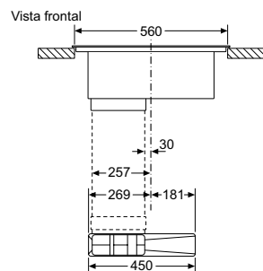
Placas combiInducción de 70 y 60 cm con extractor integrado
