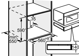
Instalación debajo de un horno compacto de 45 cm
