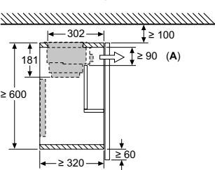
Montaje de la campana telescópica con set de alta eficiencia y marco de encastre
