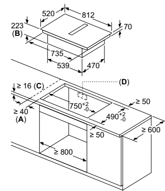
Placa flexInducción EX875LX67E de 80 cm con extractor integrado en mueble de 80 cm
