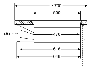
Placas flexInducción y combiInducción con extractor integrado
