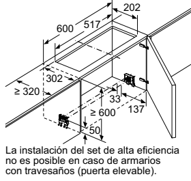
Montaje de la campana telescópica con set de alta eficiencia
