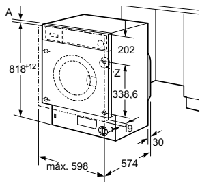
Posibilidad de colocación de la puerta del mueble con apertura hacia la derecha o izquierda
