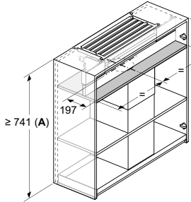
Montaje de la campana decorativa integrada con set de recirculación y prolongación de conducto, 187-360 mm
