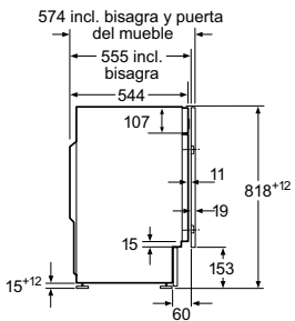
Posibilidad de colocación de la puerta del mueble con apertura hacia la derecha o izquierda
